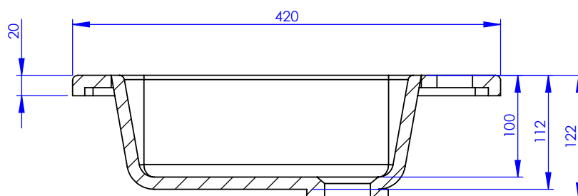
COUPE A-A
