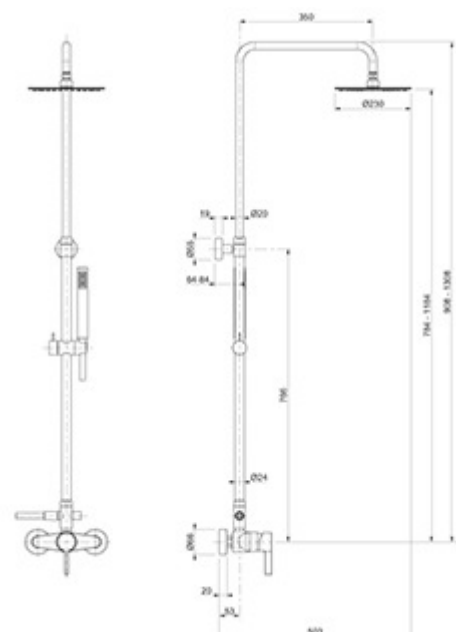
Schéma technique
