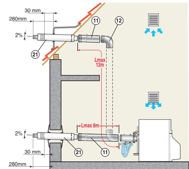
Configuration C13 - Ventouse horizontale concentrique
